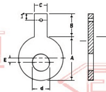
ORIFICIO EXCENTRICO E = (D-d)/2 \pm 0.01 D
